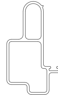
Header Z-Bar, A3606
