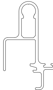
Hinge or Latch Z-Bar, A3608
