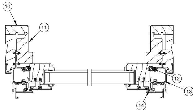
Jamb Horizontal Detail
