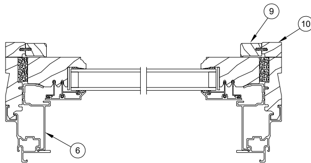
Jamb Horizontal Detail
