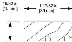
Jamb Liner, W12511
