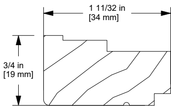
Interior Jamb Liner, W2127
