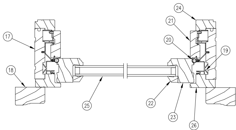
Jamb Detail
