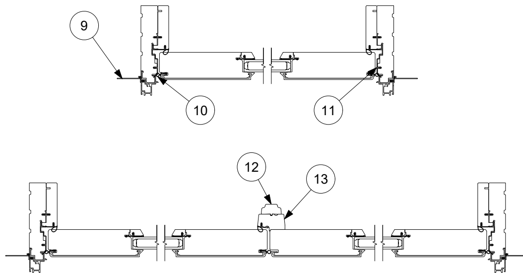
Jamb
