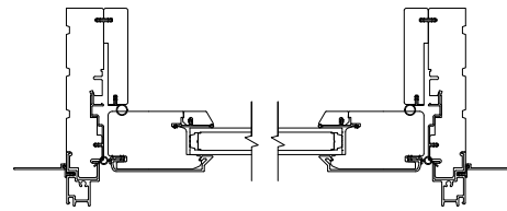
Sidelite Jamb
