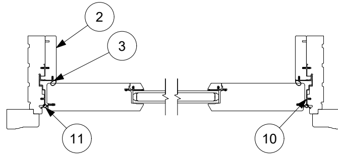
Jamb
