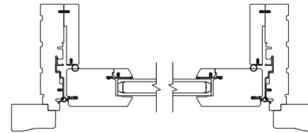
Jamb Sidelite Jamb O
