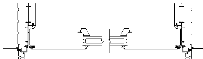
Sidelite Jamb
