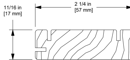
W10401 Head Jamb/Jamb Parting Stop 2 1/4 Door
