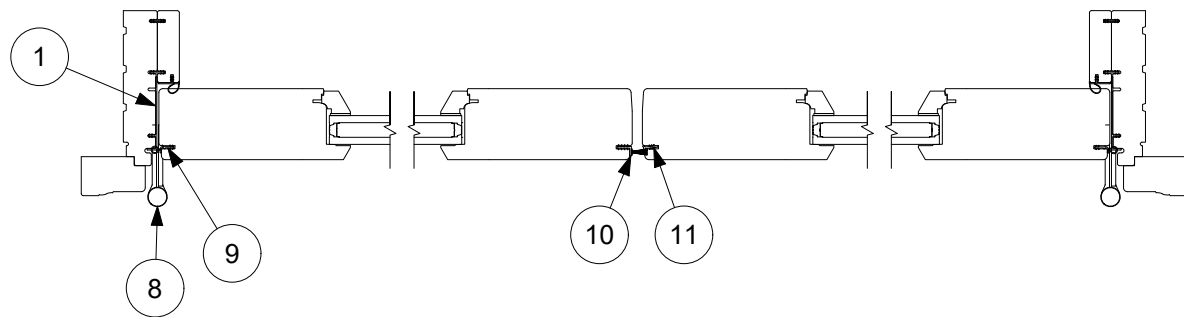
Jamb XX
