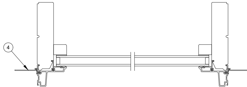
Jamb Detail
